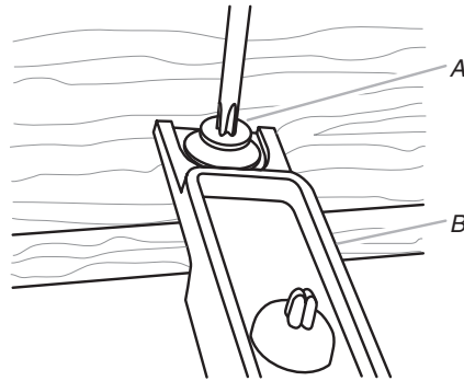
A. Door panel stud B. Installation block
