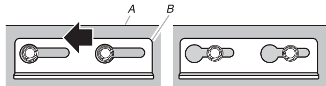
A. Door panel B. Panel top bracket
